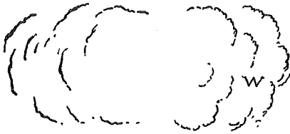
Fig. 1. Schuttrutschungen von Typ II
