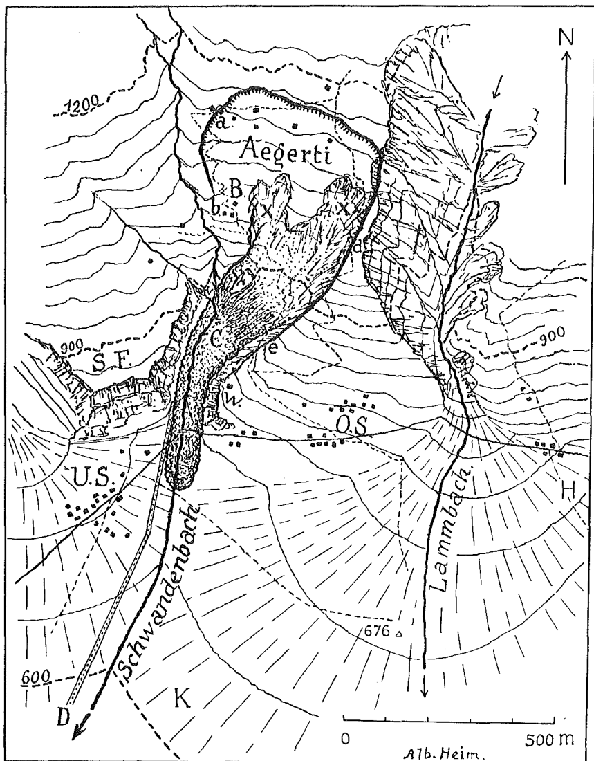
Fig. 33. Kartenskizze der Aegerti (Brienzer Kanton, Bern).
