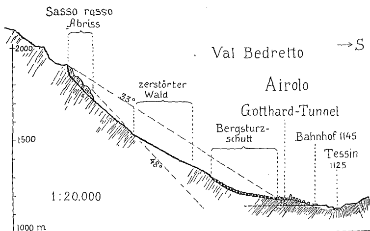
Fig. 23. Profil des Felssturzes vom Sasso rosso, Airolo.
