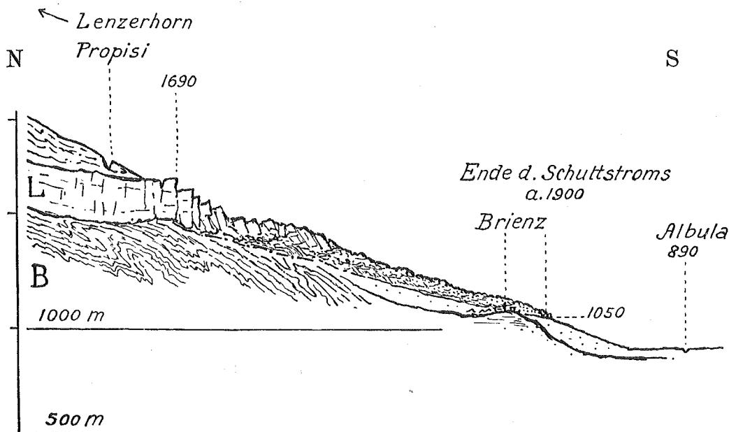
Fig. 7. Brienz (Graubünden). Seit 1878 in Bewegung. Felsbruch, abfliessend als Schleichstrom (Typus XII).
