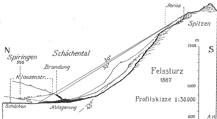
Fig. 24. Felssturz ab den Spitzten bei Spiringen, Schächental.
